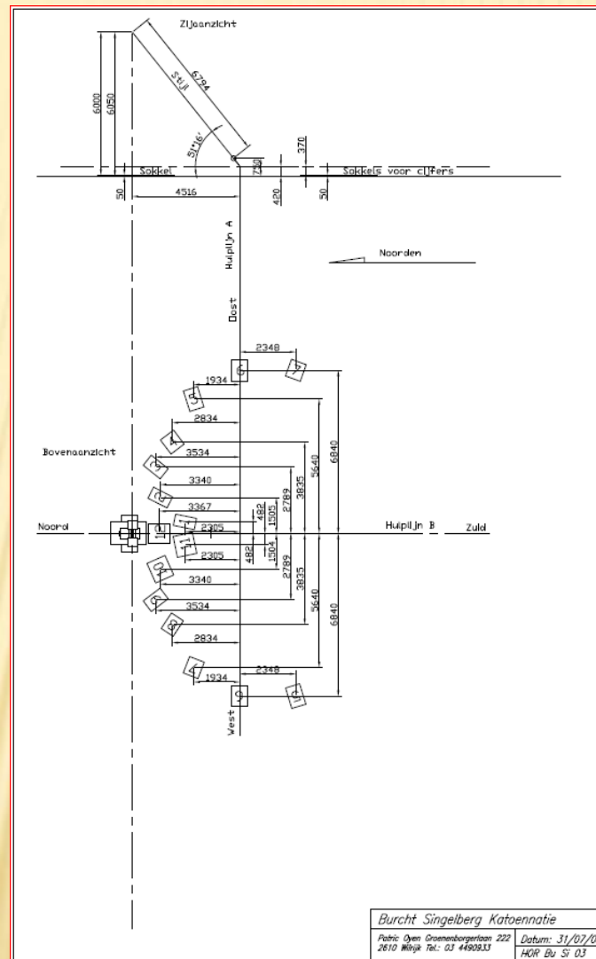
Ontwerptekening met maten P. Oyen
